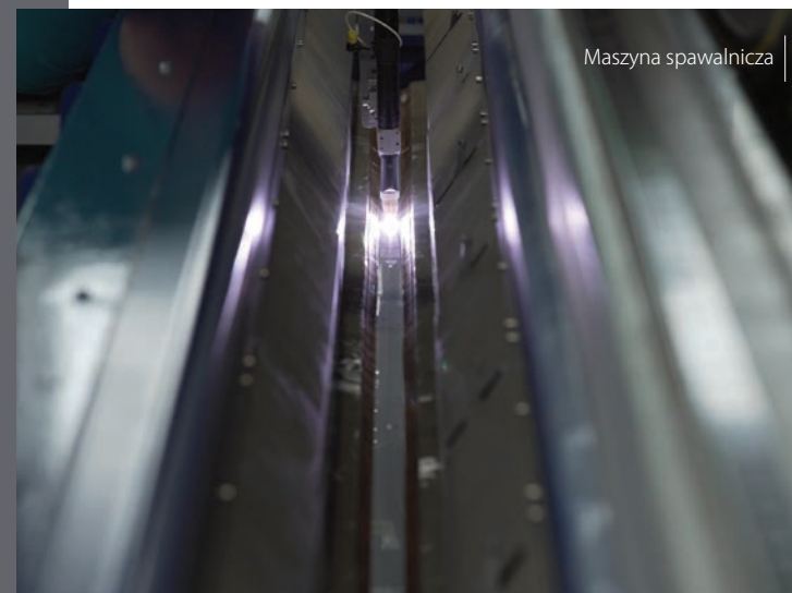
Robot spawający
